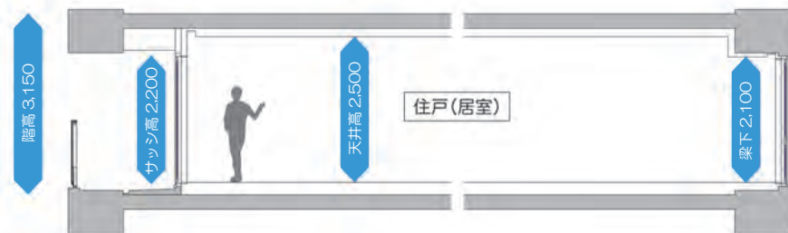
■住戸断面図の例
