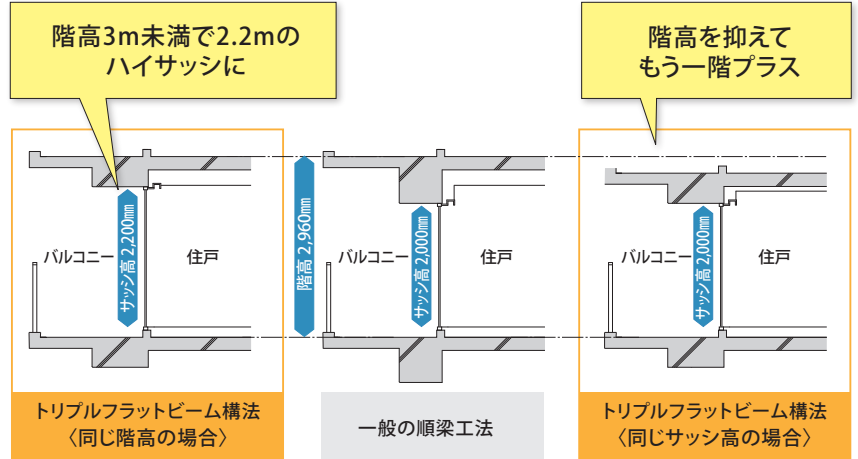
■構法の違いによる断面比較
