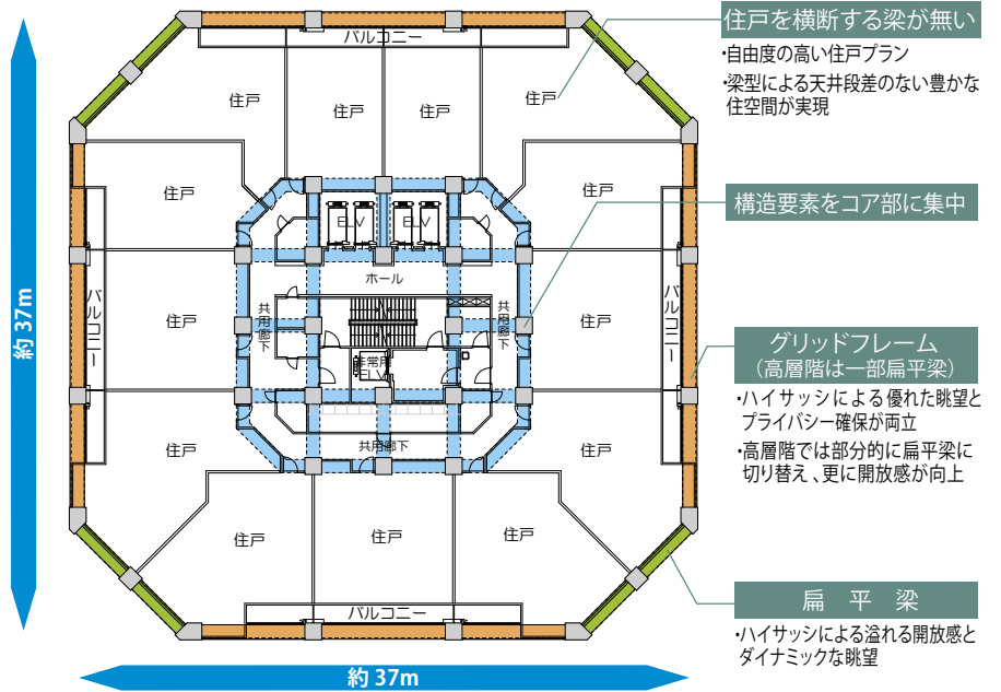
■住戸断面の例(扁平梁部)
