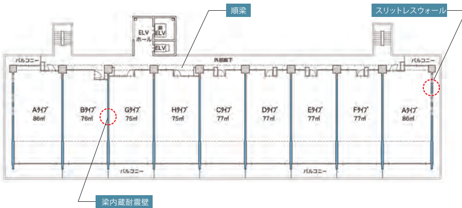
■基準階平面図の例
