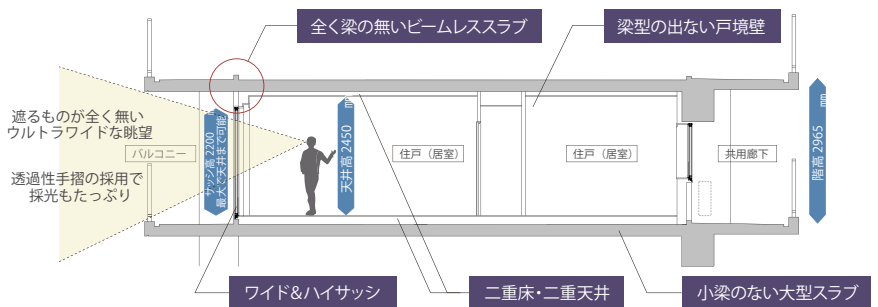
■住戸断面の例
