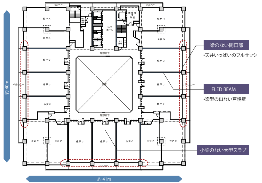
■住棟基準階 平面図の例
