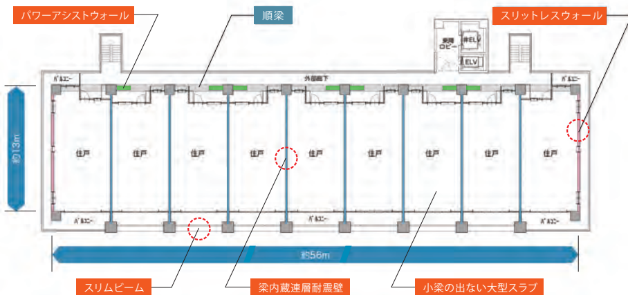
■基準階平面図の例
