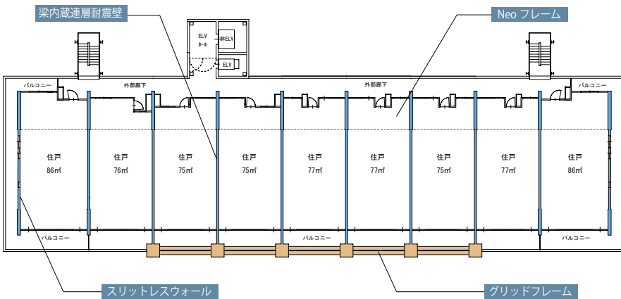
■基準階平面図の例
