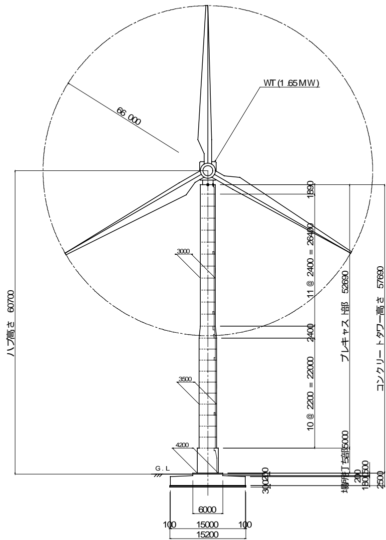
正面図
