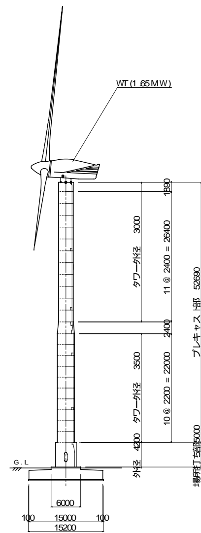
側面図
